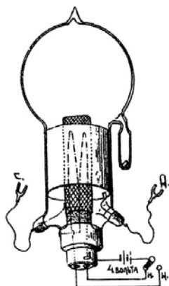
Рис. 2. Конструкция лампы Папалекси. Ручной подпоручица Магнусовского, 1917 г.
